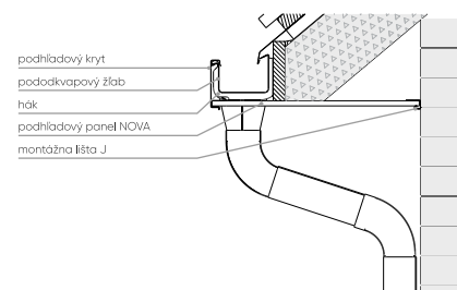
Priečny rez znázorňujúci montáž na streche s odkvapom
