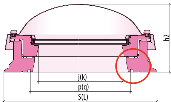
XRD XRD/W
